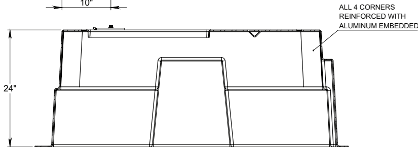
SECCIÓN S-S ESCALA 1 : 13
