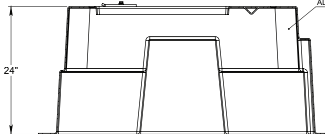
SECCIÓN S-S ESCALA 1 : 13
